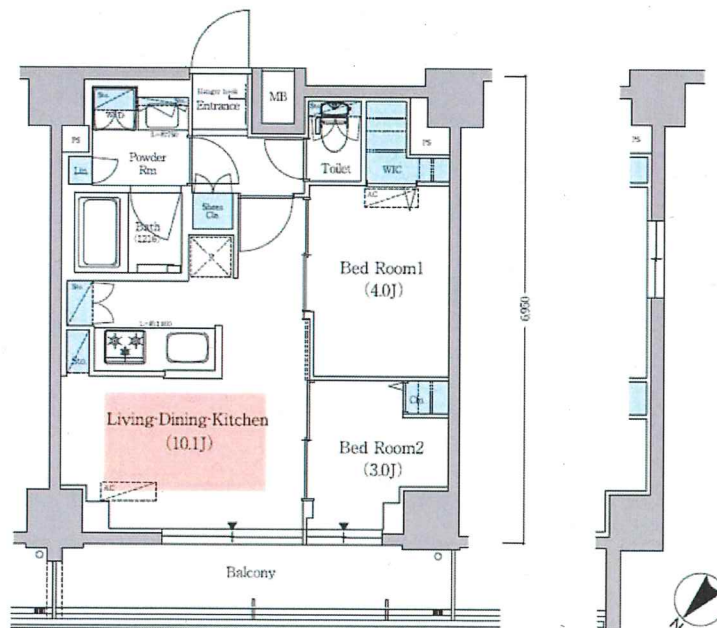
801-901号室部分図
